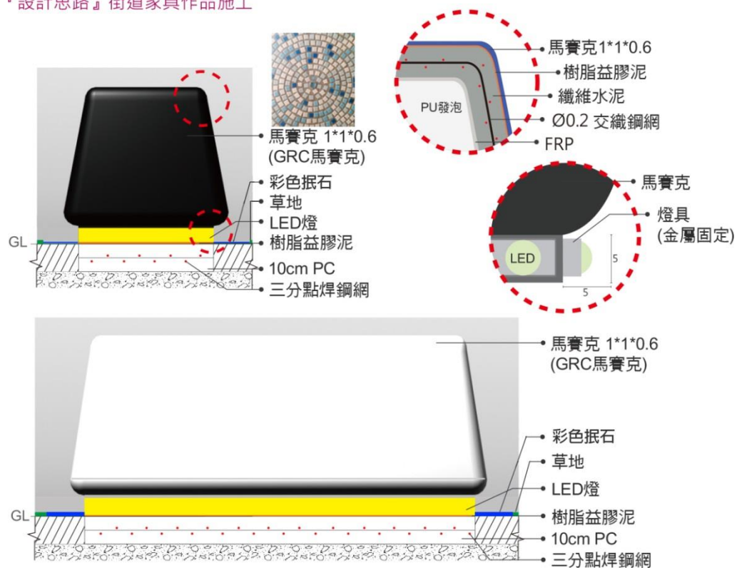
實體作品施作圖說
